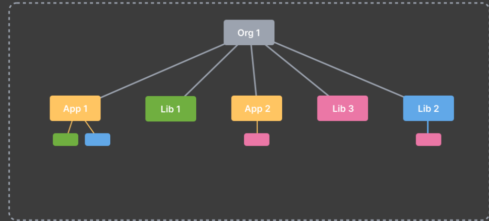
Monorepo
