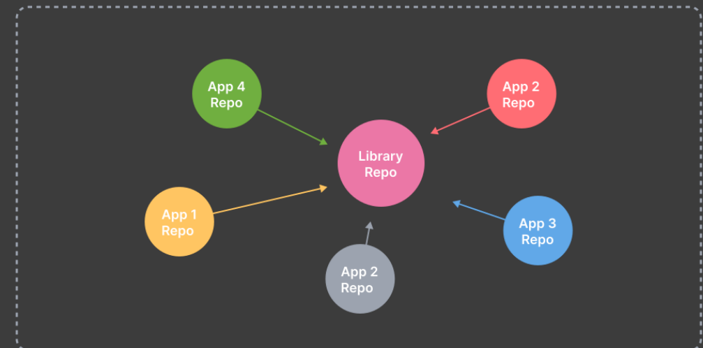
Polyrepo
